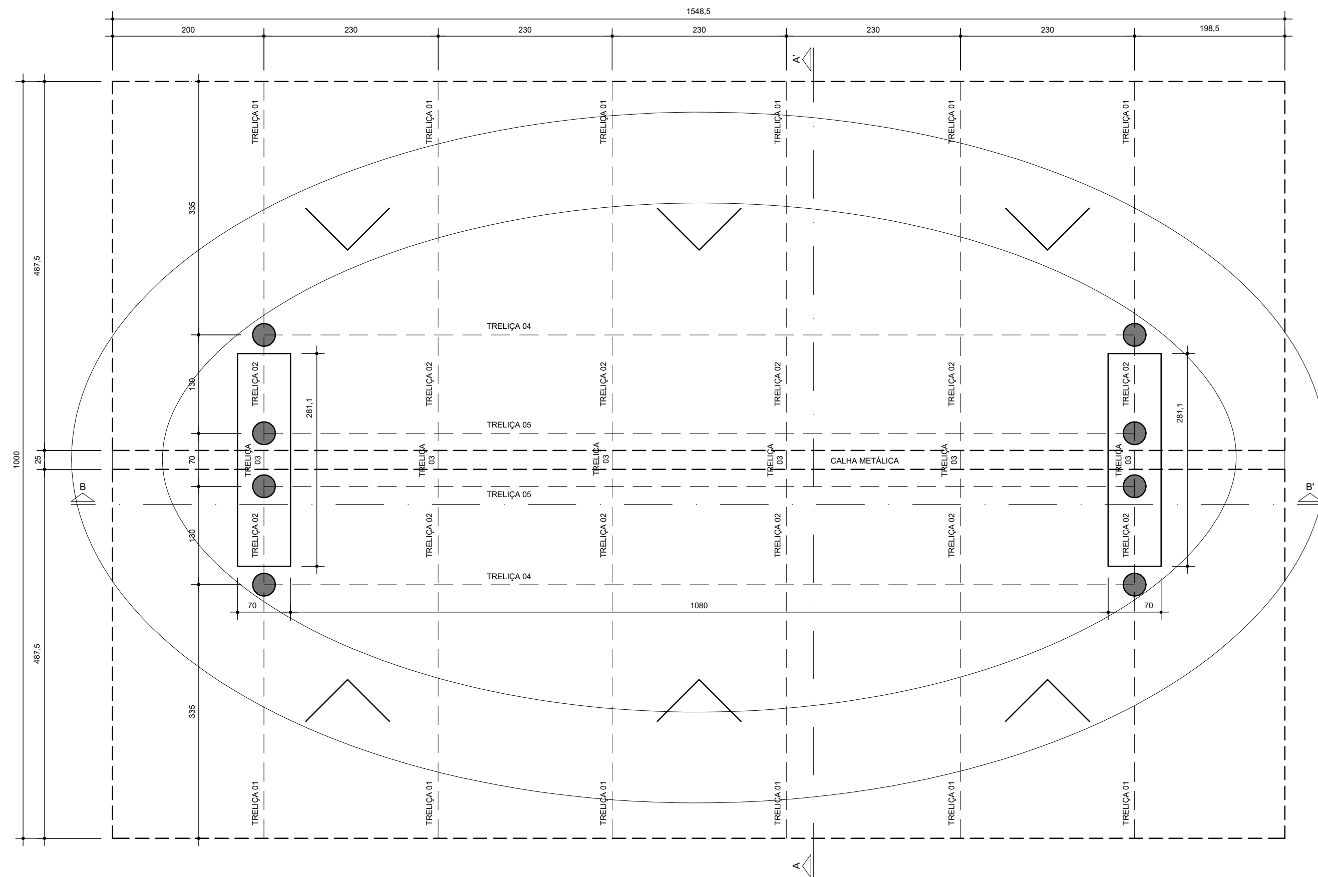
PLANTA BAIXA/COBERTURA Esc: 1/50
