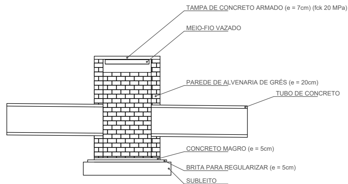
CORTE B-B' – CAIXA BL
